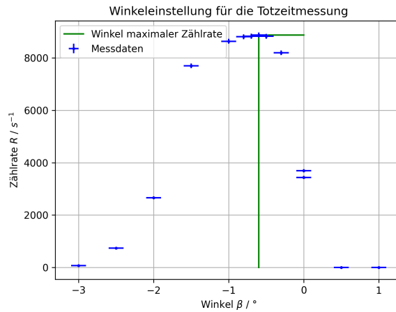
Abbildung 19: Bestimmung des Winkels \beta der maximalen Zählrate R für die Totzeitmessung (Messwerte: Tabelle 20)
