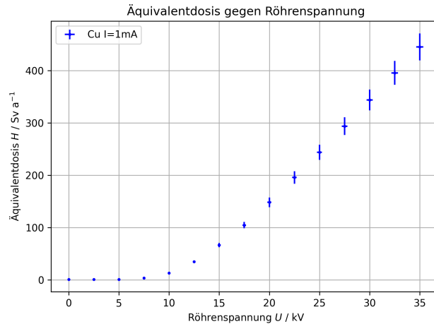
Abbildung 15: Äquivalentdosis H pro Jahr in Abhängigkeit der Röhrenspannung U (Kupfer-Röhre, I = 1 mA)
