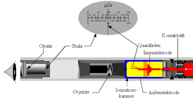
Abbildung 5: Aufbau des Stabdosimeters [4]
