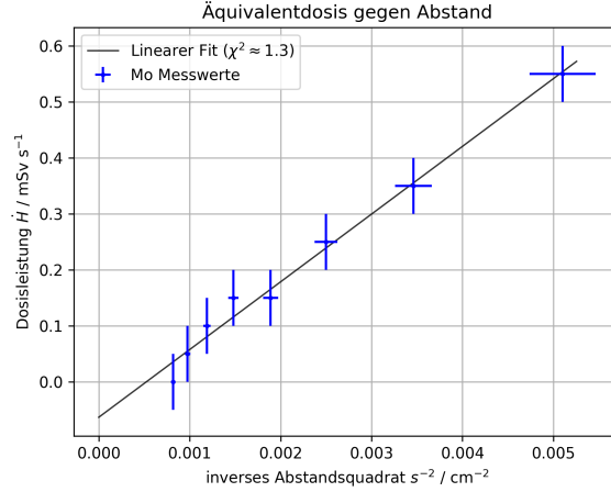
Abbildung 18: Linearer Fit der Äquivalentdosis H über Integrationszeit \Delta t = 2 s gegen inverses Abstandsquadrat s^{-2} (Molybdän-Röhre, I = 0,2 mA, U = 35 kV)
