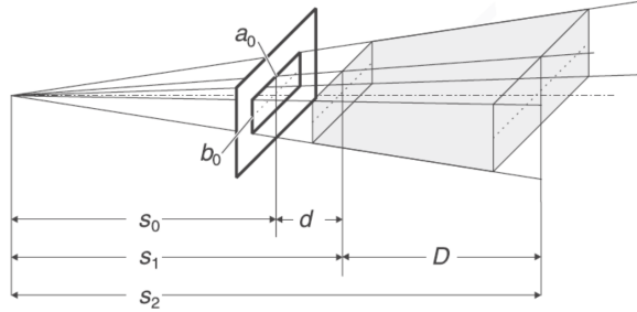
Abbildung 7: Dimensionen des durchstrahlten Volumens im Plattenkondensators [7]
