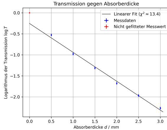
Abbildung 22: Linearer Fit des Logarithmus des Transmissionsgrads \log T gegen Absorberdicke d (Molybdän-Röhre, U = 35 kV, ohne Zirkoniumfilter)
