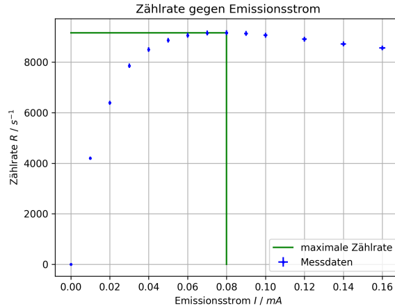
Abbildung 20: Zählrate R gegen Emissionsstrom I (Kupfer-Röhre, U = 35 \text{ kV} )
