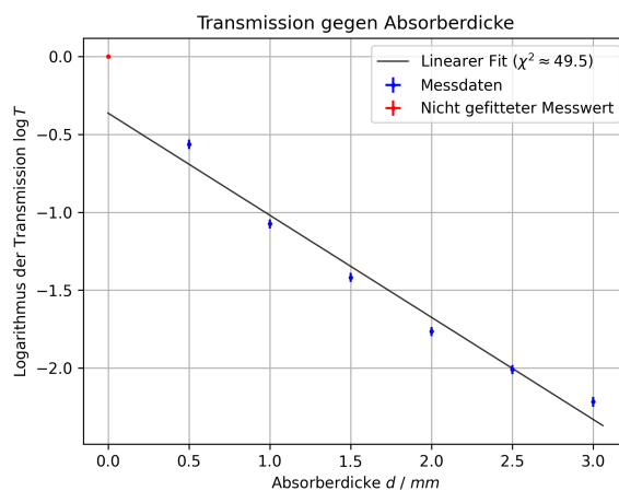
Abbildung 23: Logarithmus des Transmissionsgrads \log T gegen Absorberdicke d (Molybdän-Röhre, U = 35 kV, mit Zirkoniumfilter)
