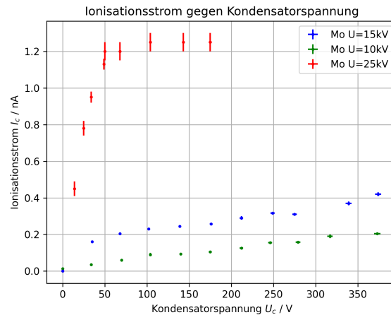
Abbildung 9: Ionisationsstrom I_C des Kondensators in Abhängigkeit der Kondensatorspannung U_C für drei verschiedene Röhrensparnungen (Molybdän-Röhre, I = 1\text{ mA} )
