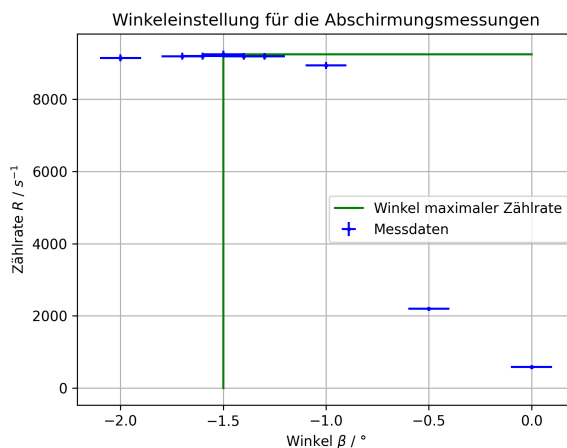
Abbildung 21: Bestimmung des Winkels \beta der maximalen Zählrate R für die Abschirmungsmessungen (Messwerte: Tabelle 22)
