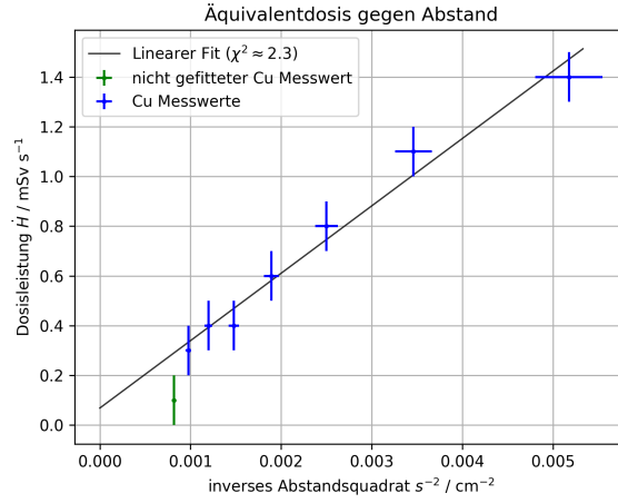
Abbildung 17: Linearer Fit der Dosisleistung \dot{H} über Integrationszeit \Delta t = 1 s gegen inverses Abstandsquadrat s^{-2} (Kupfer-Röhre, I = 0,1 mA, U = 35 kV)
