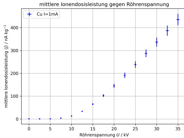
Abbildung 13: mittlere Ionendosisleistung \langle j \rangle in Abhängigkeit der Röhrenspannung U (Kupfer-Röhre, I = 1 \text{ mA} )
